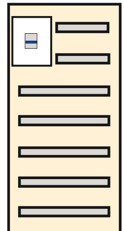
DIN/7 & DINS/7 2x12+5x24 = 144 mód.+ICP
