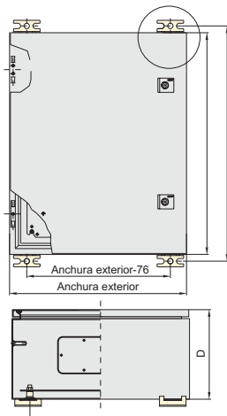
Dimensiones de los cuadros
