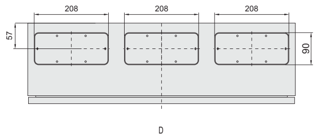
Dimensiones de las placas de montaje
