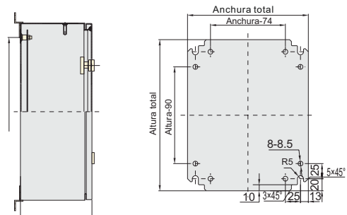
Dimensiones de las placas de montaje
