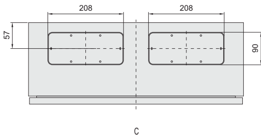
Dimensiones de los cuadros
